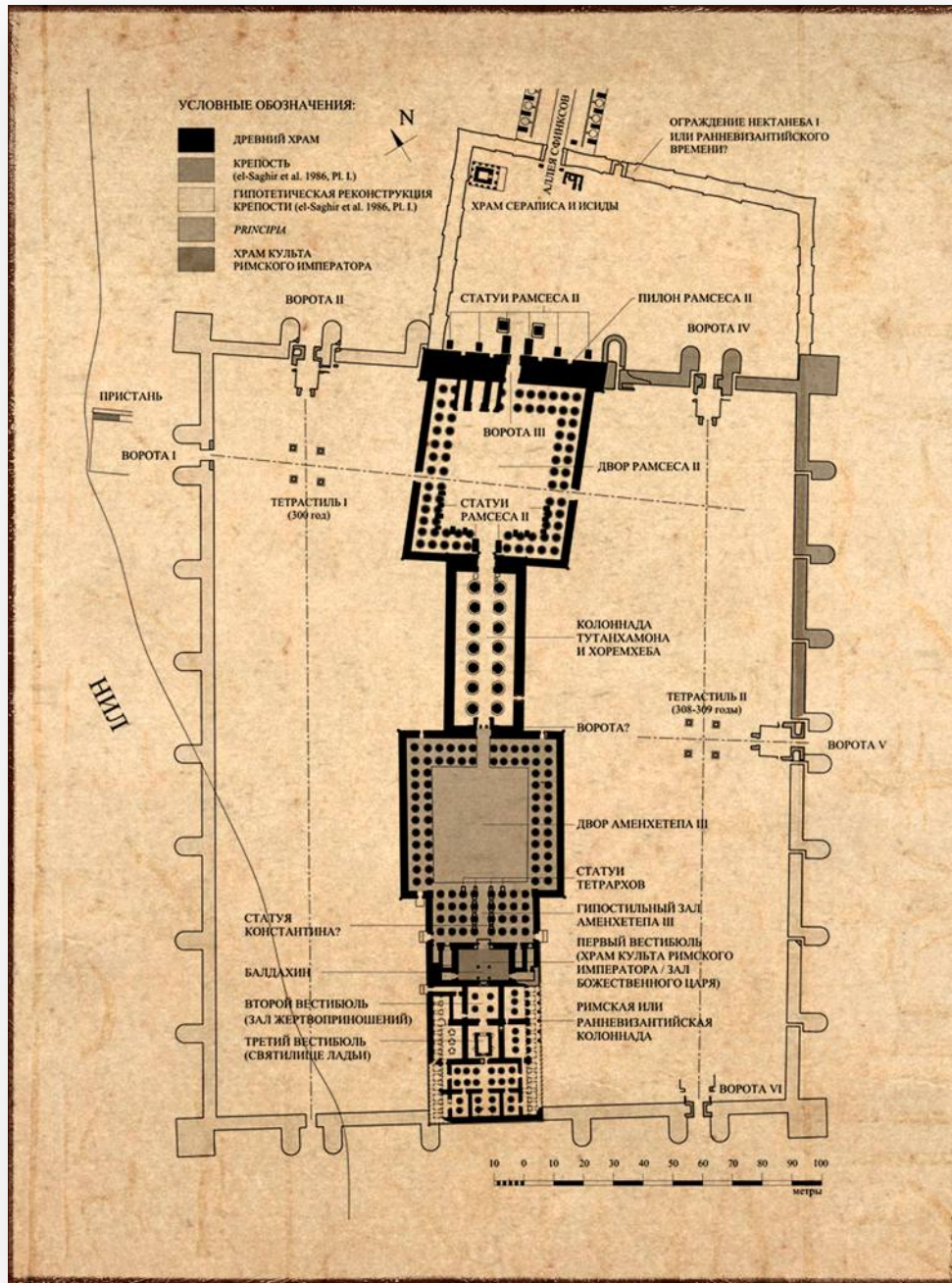
План римской крепости в Луксоре Начерчено Д.А.Карелин на основании: el-Saghir et al 1986. Pl. 1; Bell 1997. Fig. 56
